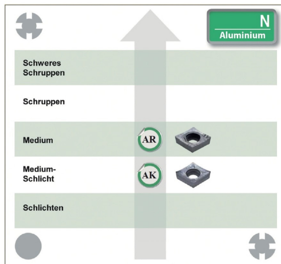
Spanbrecher für positive Wendeplatten
