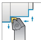
Rechtsausführung 95°
