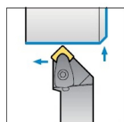
Rechtsausführung 45°
