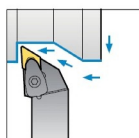
Rechtsausführung 93°
